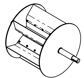
Rotor PP450-710
